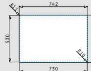
Montáž do roviny
