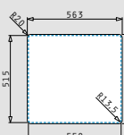
Montáž do roviny
